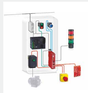
Controllo protezione mobile con arresto emergenza in SIL3, PL=E
