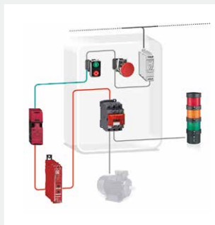
Controllo protezione mobile in SIL1, PL=C
