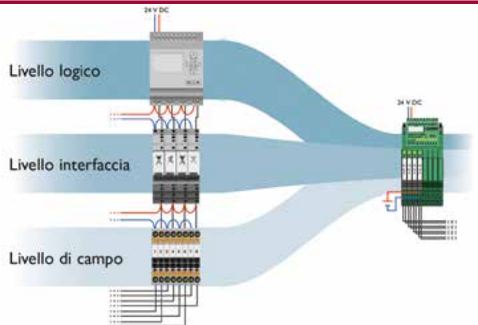
CABLAGGIO TRADIZIONALE
